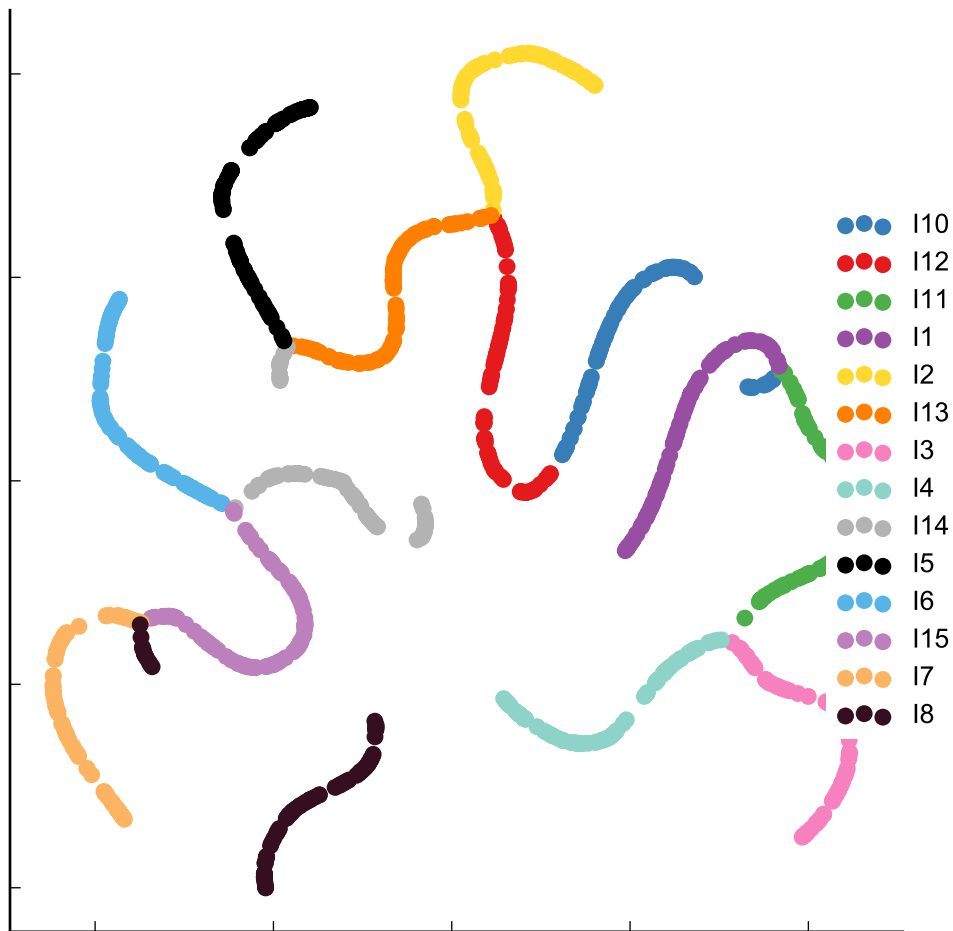
t-SNE
